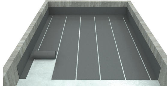
04_ 탄소저감시트 부착(바닥)
