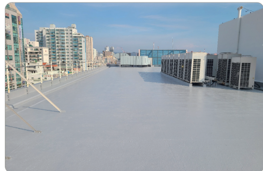
시공완료
